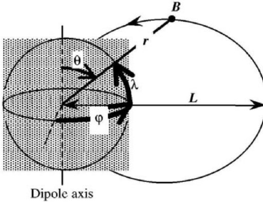
Fig. 6. Magnetic coordinates
